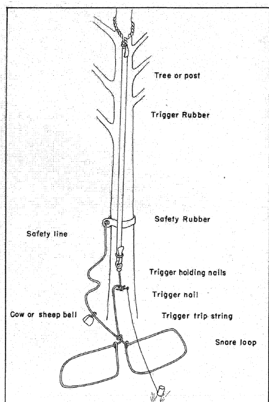
FIGURE 1. "Improved Deer Snare", showing details of construction. Drawing by Cliffo Corson. Figura 8.8: disegno originale del laccio a elastico per la cattura di ungulati del 1957.
